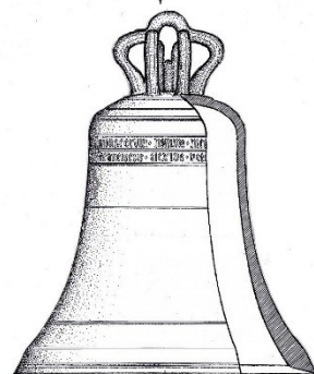
CAMPANA II LAB 3 Ømm 1007 Kg 700 MCCCCXXIII
