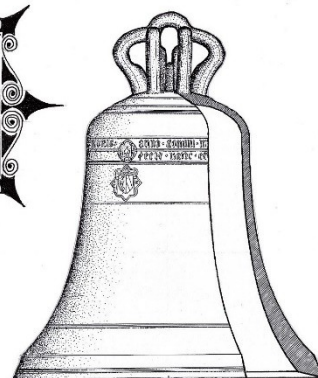
CAMPANA I SOL 3 Ømm 1125 Kg 950 MCCCCXXIII
