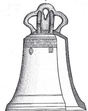
CAMPANA III LAB 3 Ømm 973 Kg 600 MCCCCXXXVIII
