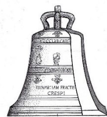
CAMPANA IV DO 4 Ømm 738 Kg 240 MDCCLV
